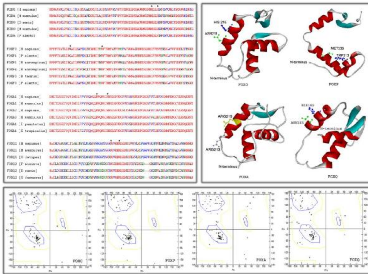
图 4 FOX 家族保守区域比对及三级结构建模
