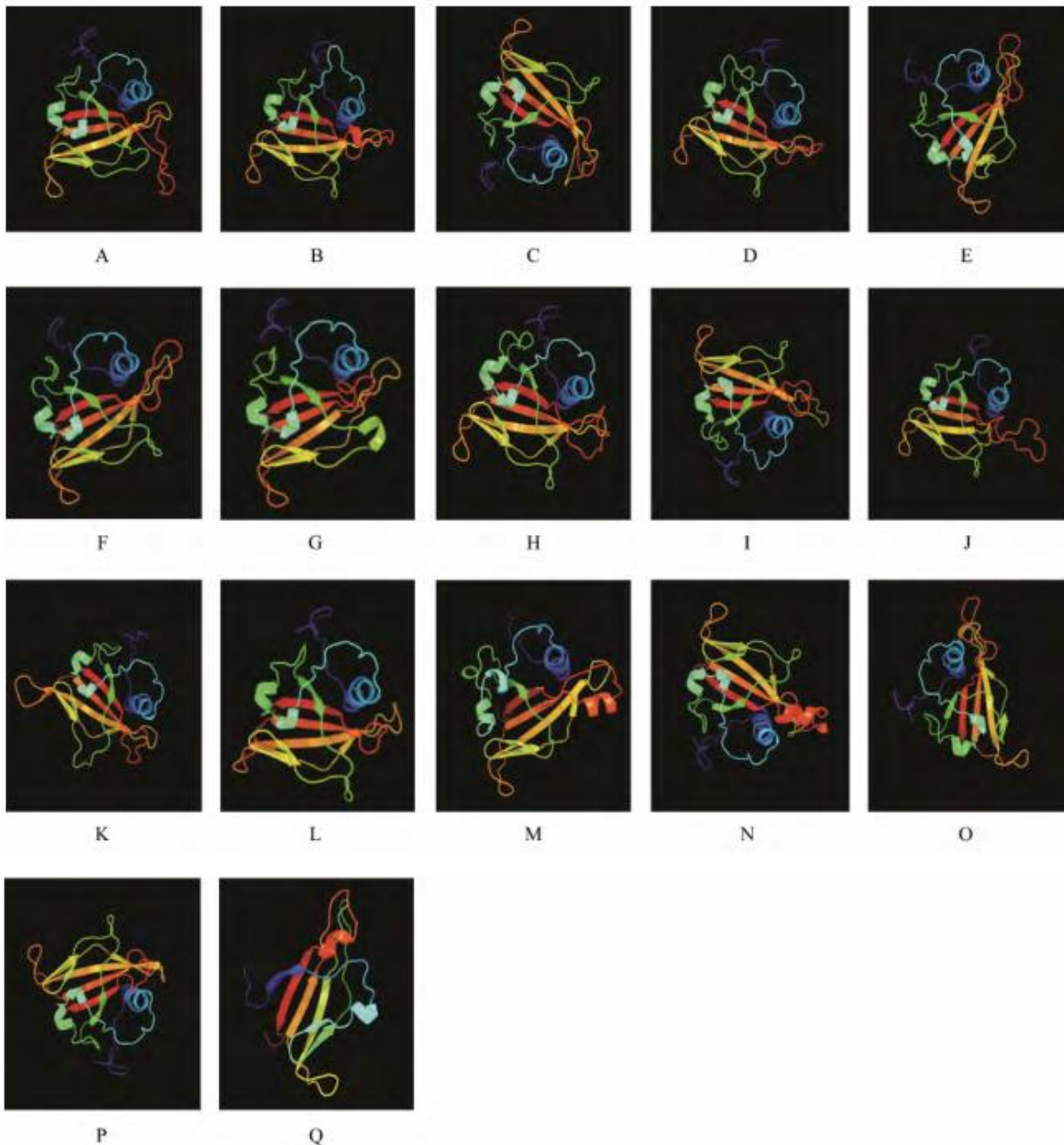
图 3 17 个代表性的毛竹 NAC 蛋白质三级结构
