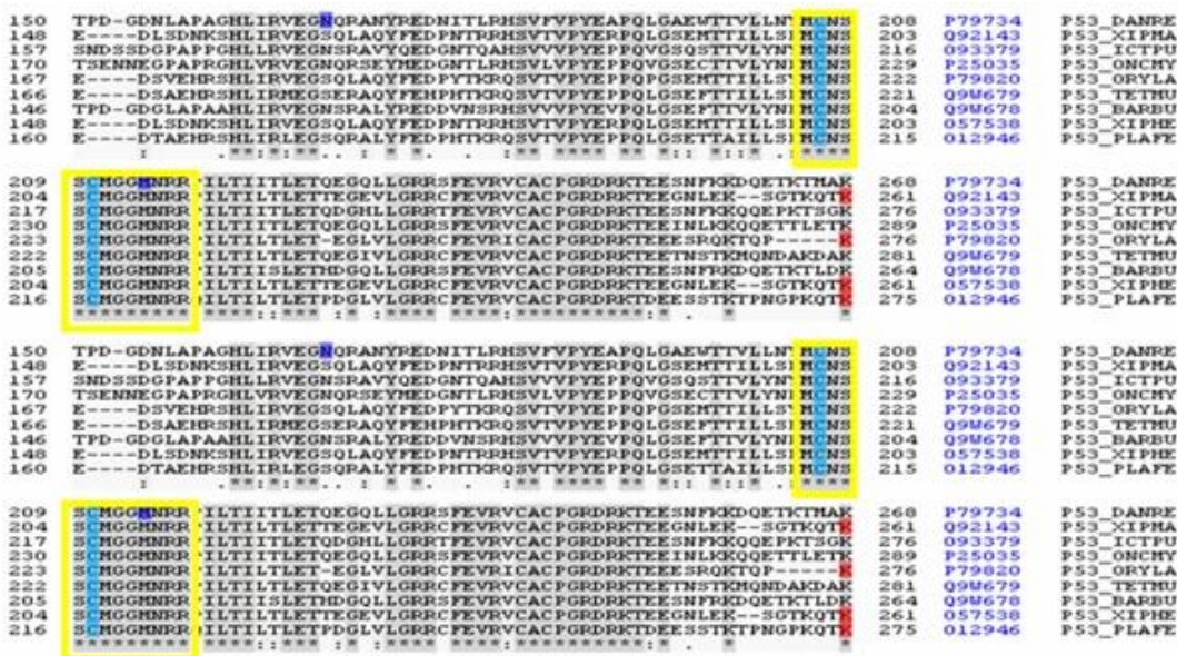
图 1 MSA 的 snapsort. 这里, "*"表示比对所有序列相同; "."表示保守取代; "."表示半保守. 红色表示主题; 深灰色表示相似性; 浅蓝色表示金属结合; 紫色表示诱变. 所选择的保守区域由黄色框突出显示
